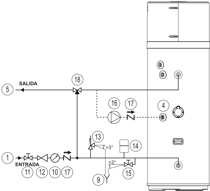
fig. 16 - Ejemplo de sistema de agua
