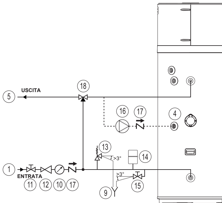
fig. 16 - Esempio impianto idrico
