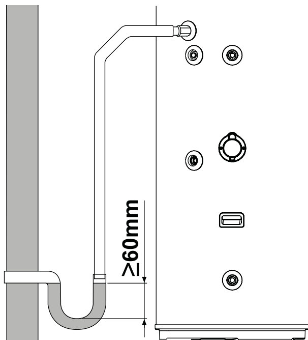
fig. 17 - Esempi di collegamento di scarico della condensa attraverso un pozzetto di intercettazione
